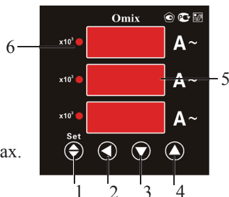
Рис. 1 – Управляющие элементы
